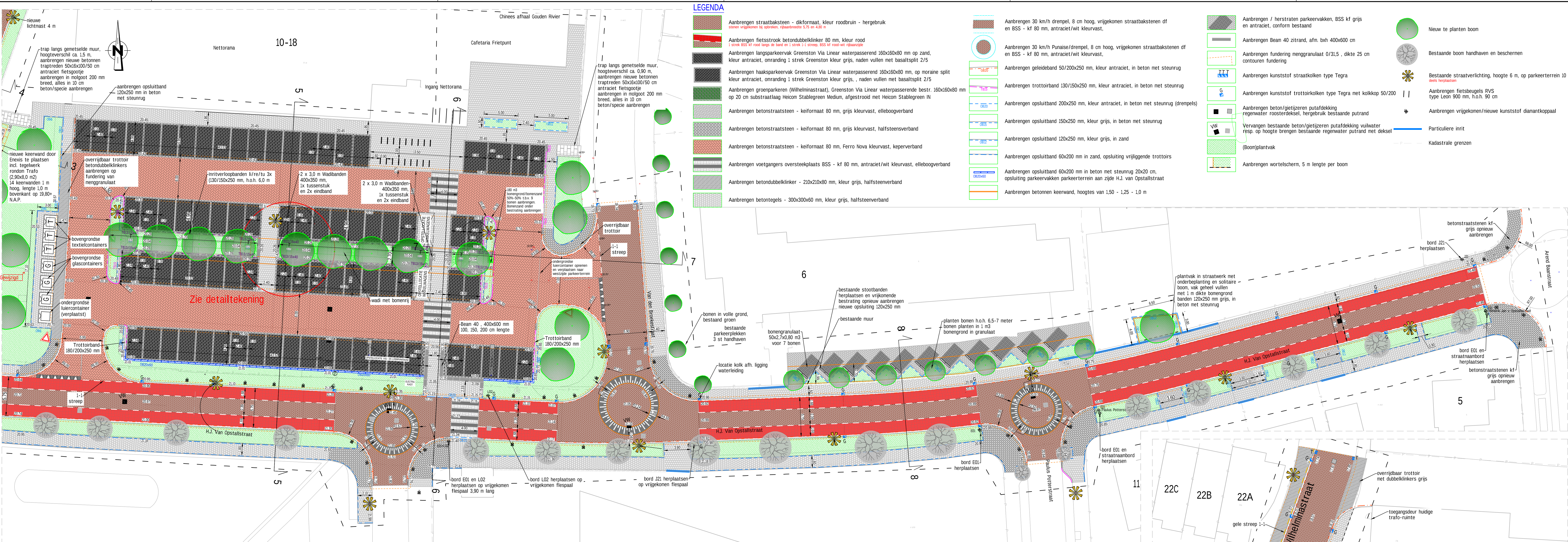
Bovenaanzicht nieuwe verhardingen en groen, deel oost Wilhelminastraat-Arend Baanstraat (schaal 1:200)
